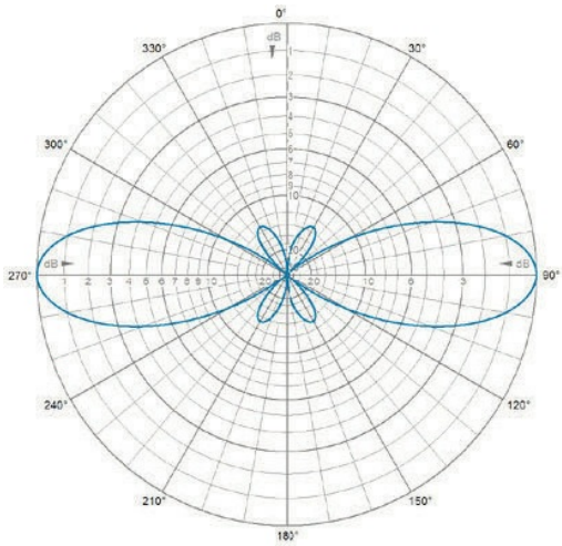
E-Plane | 445 MHz
