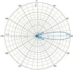
E-Plane | 425 MHz
