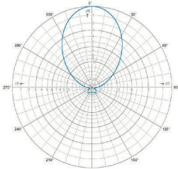
H-Plane | 425 MHz
